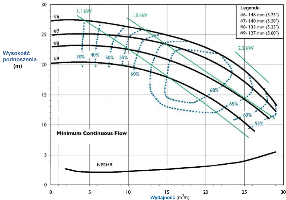
DB15 WYDAJNOŚĆ 2900 RPM
