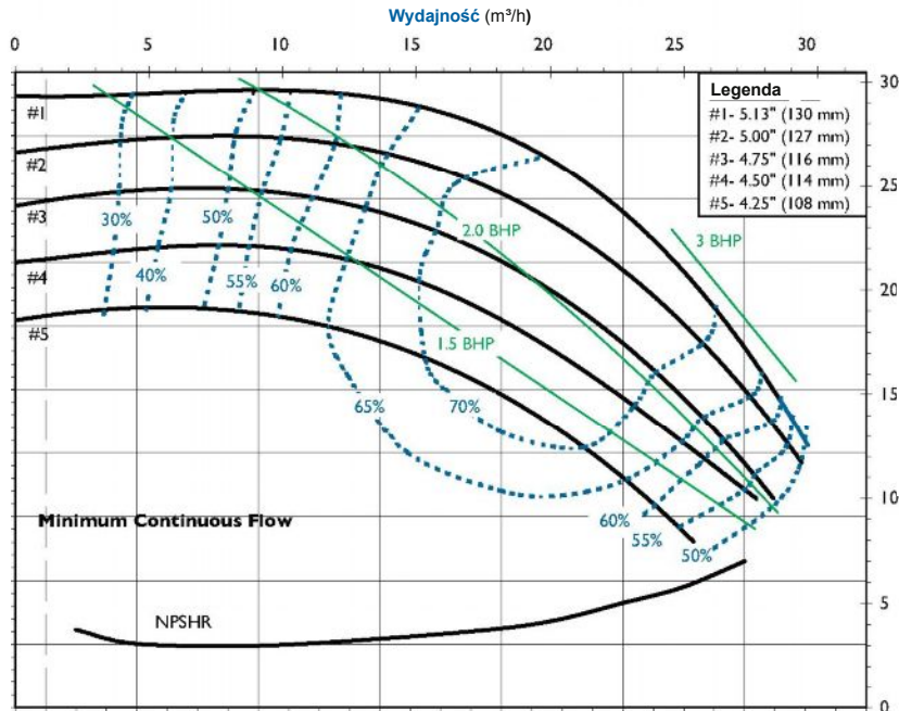
DB15 WYDAJNOŚĆ 3450 RPM
